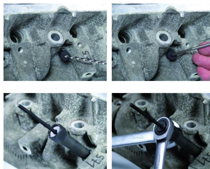
C2087 CONJUNTO PARA LA EXTRACCIÓN DE LAS MECHAS DE LOS CALENTADORES ROTOS M8 Y M10 159 €
